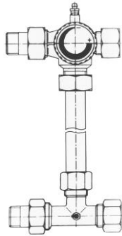
Kurzschlußstrecke
